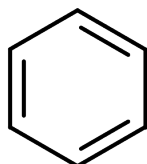
cyclohexa-1,3,5-triene (Kekulé)
