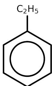
ethylbenzene
