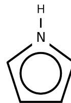
pyrrole
