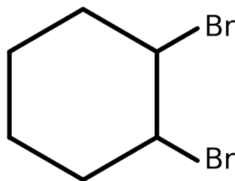
1,2-dibromocyclohexane
