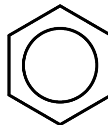
benzene
